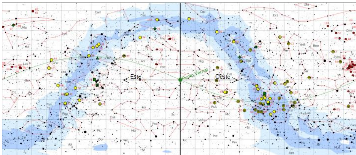
Gráfico 1 - Mapa de estrellas que muestra vectores de direcciones celestes (este/oeste) en relación con el punto vernal (en el centro)
