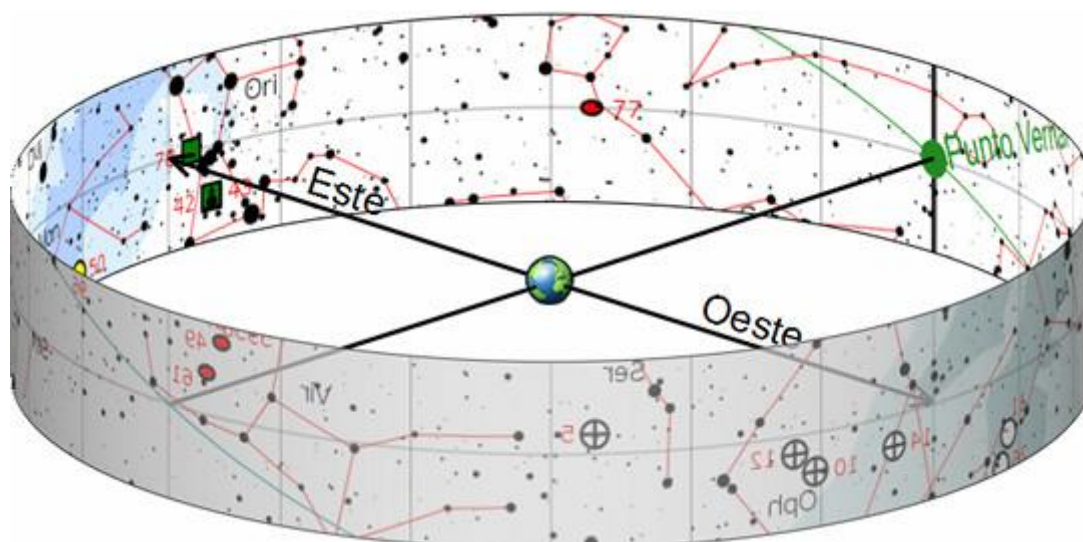
Gráfico 2 - Visualización de vectores de direcciones celestes (rango: \pm 10^\circ de declinación)
