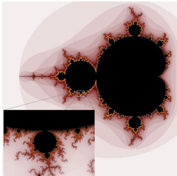
Figura 2 – Ilustración de la autosimilaridad de los fractales
